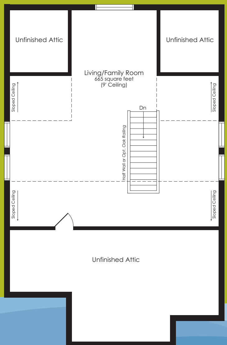
Optional Loft
